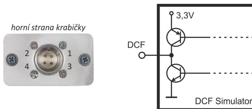
obr. 6 – zapojení konektoru a náčrtek zapojení DCF výstupu
