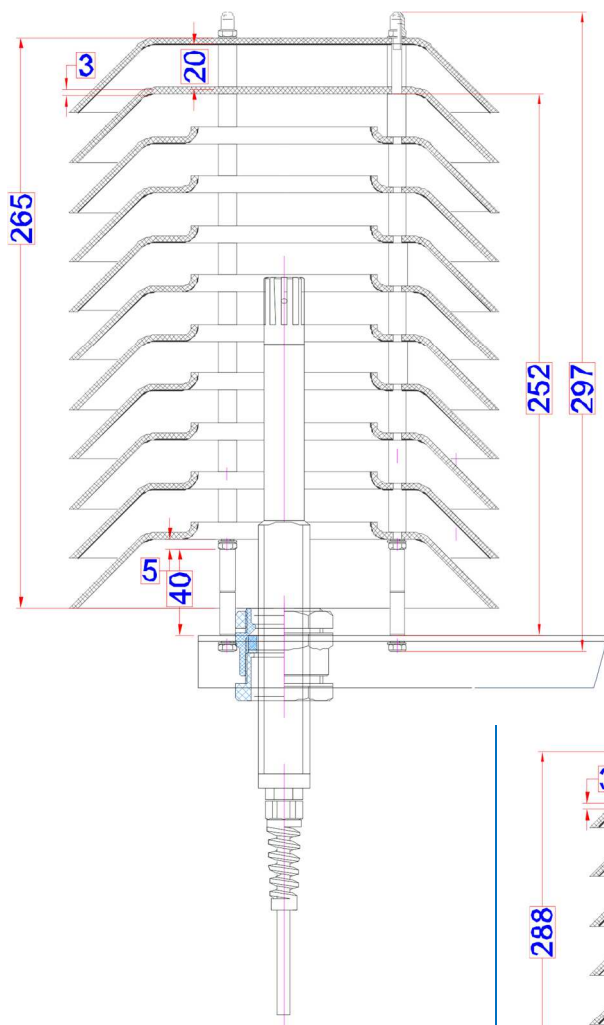
OAR-961_V Dedykowany czujnik HMP155
